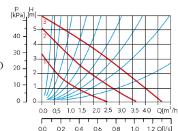
W0202 Oběhová čerpadla FERRO pro pitnou vodu
